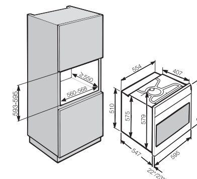
Vestavná pečicí trouba H 2465 B/BP, H 2467 B/BP, H 2861 B/BP, H 2766 B/BP
