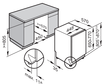
Myčka nádobí G 5481 SCVi
