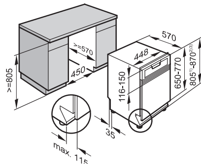
Myčka nádobí G 5430 SCi
