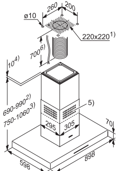
Ostrovňový odsavač par PUR 98 D
