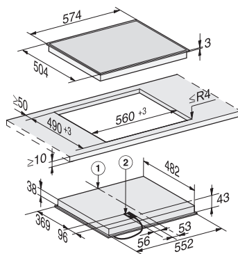
Sklokeramická varná deska KM 6520 FR
