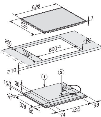
Indukční varná deska KM 7564 FR
