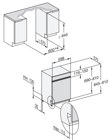
Myčka nádobí G 5215 Sci XXL
