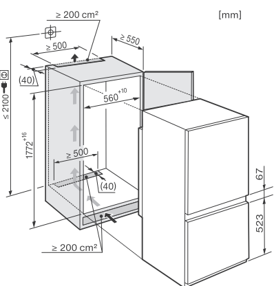
Vestavná chladnička s mrazničkou KF 7731 E
