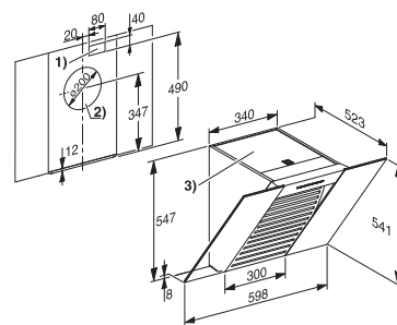
Nástěnný odsavač par DA 6066 W Black Wing / White Wing
