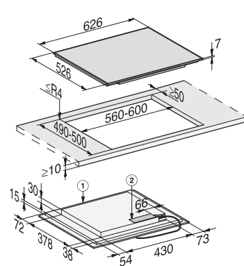
Indukční varná deska KM 7464 FR
