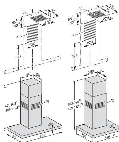
Nástěnný odsavač par DAW 1920 / DAW 1620
