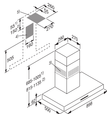
Nástěnný odsavač par PUR 98 W
