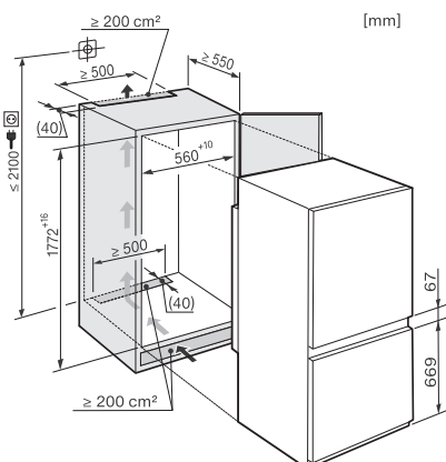
Vestavná chladnička s mrazničkou KFN 7733 F
