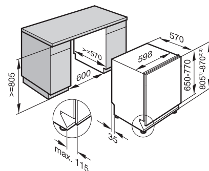
Myčka nádobí G 5260 SCVi G 5050 SCVi
