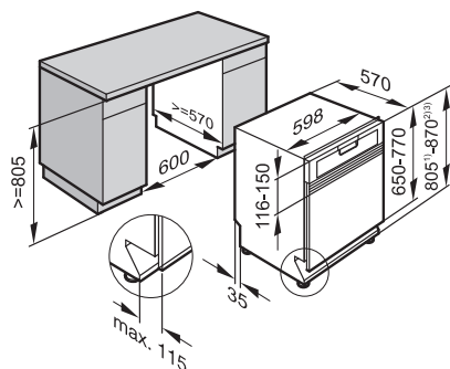
Myčka nádobí G 5210 SCi G 5000 SCi
